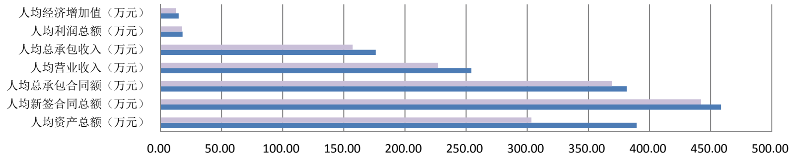
图1-2 2018年电力勘测设计行业人均指标与2017年对比图
