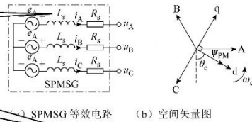
图 2 SPMSG 等效电路和空间矢量图
